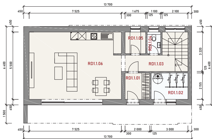
PÔDORYS PRÍZEMIA
