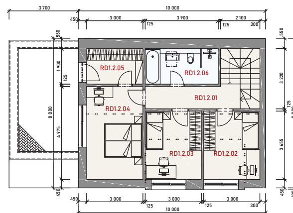
PÔDORYS PODKROVIA
